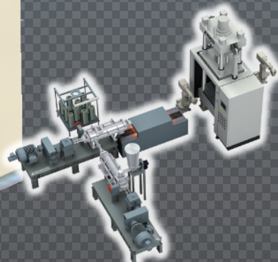
Carbon-LFTDシステム
